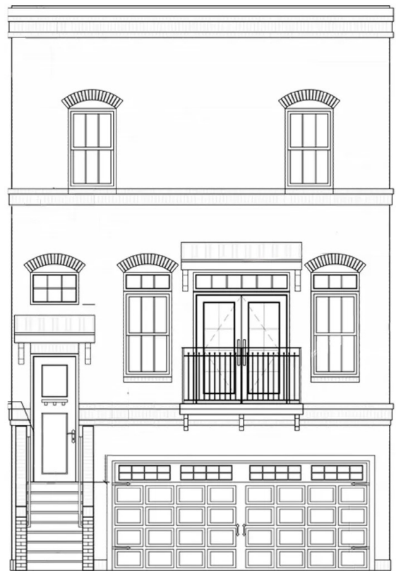
ELEVATION B
